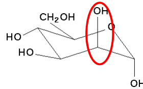
\alpha -D-Mannosio
