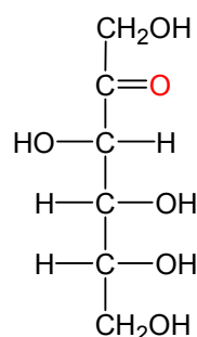
D-fructose
